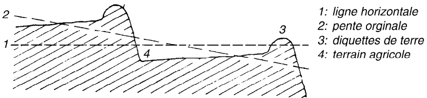
Figure 26 : Terrasse d'absorption.
