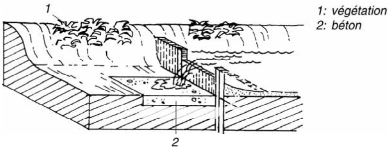
Figure 31 : Stabilisation d'une ravine.
