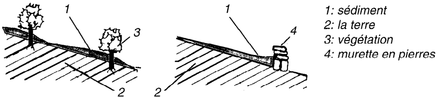
Figure 22 : Formation d'une terrasse à l'aide d'une ligne de végétation ou d'une murette en pierres.
