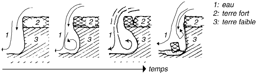
Figure 32 : Extension rétrograde.
