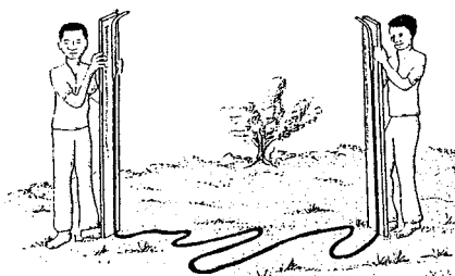
Figure 37 : Niveau d'eau.
