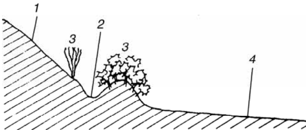
Figure 28 : Terrasse de dérivation.
