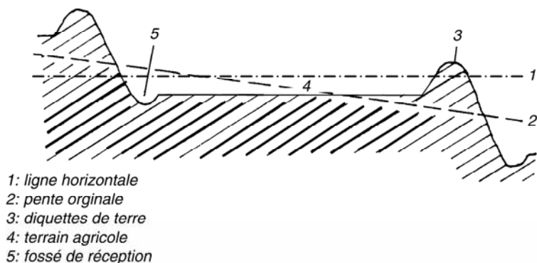
Figure 21 : Construction d'une terrasse.
