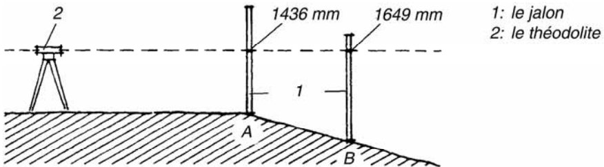
Figure 36 : Nivellement à l'aide du théodolite.
