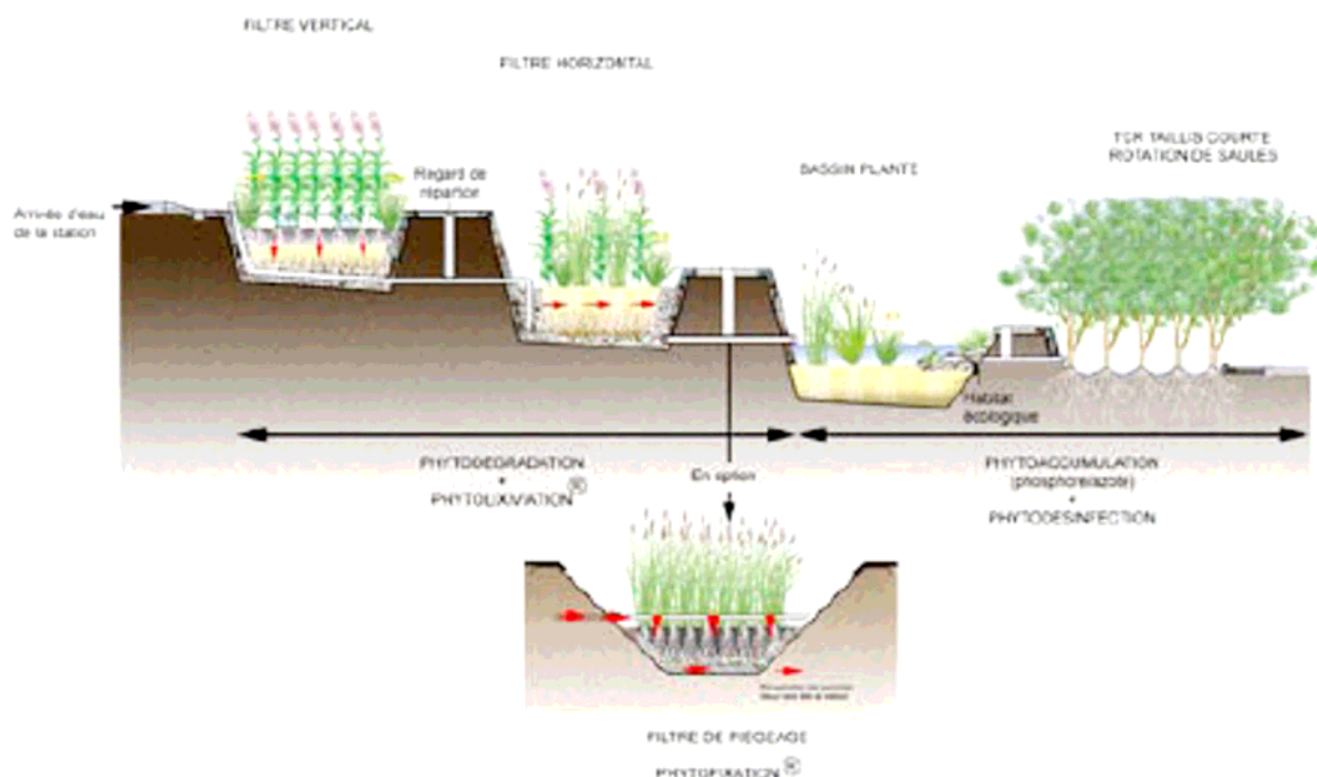
Graphique n° 19. Schéma d'un jardin filtrant pour le traitement des eaux (source : Phytostore, www.phytostore.com )
