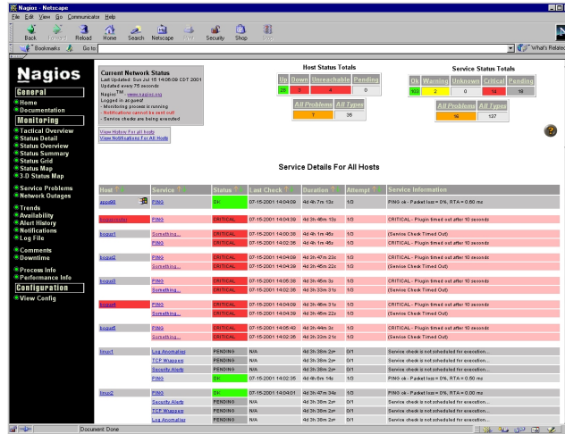
FIG. 5 – Nagios - Liste des états des services supervisés.
