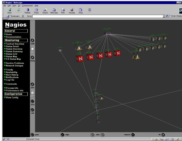
FIG. 7 – Nagios - Représentation graphique des machines supervisées.
