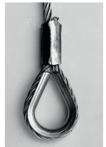
« Œil sur cosse et manchon sertis : montage réservé au câble souple ou extra-souple.
