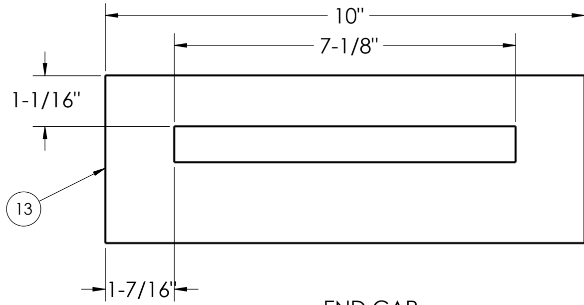
END CAP
