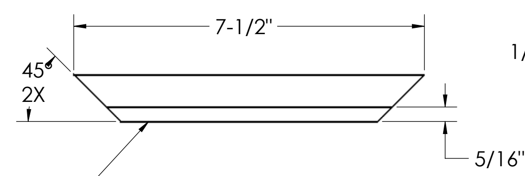
DOOR FRAME END
