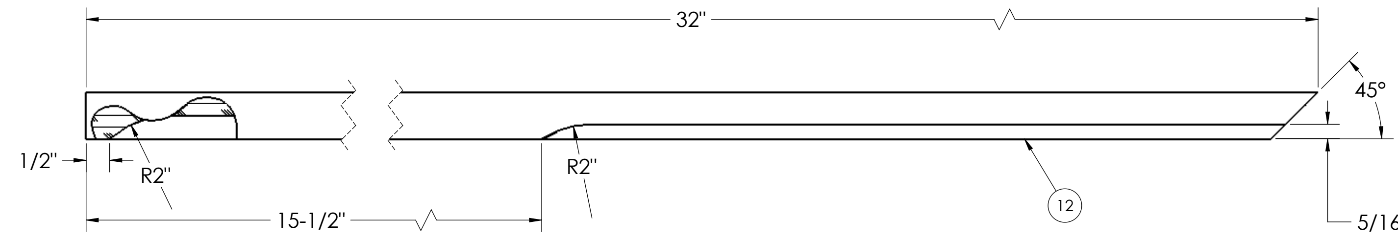
DOOR FRAME LOWER
