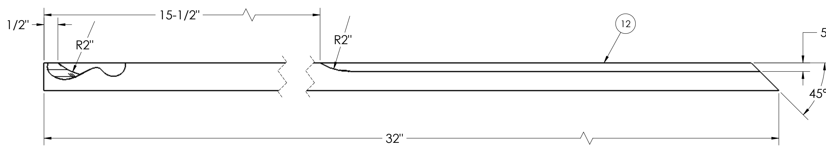
DOOR FRAME UPPER
