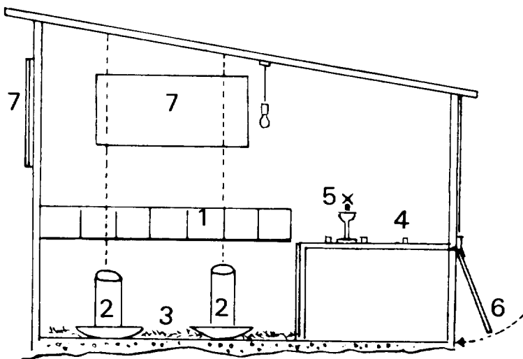
Figure 2. INTÉRIEUR DU POULLAILLER VU DE PROFIL
