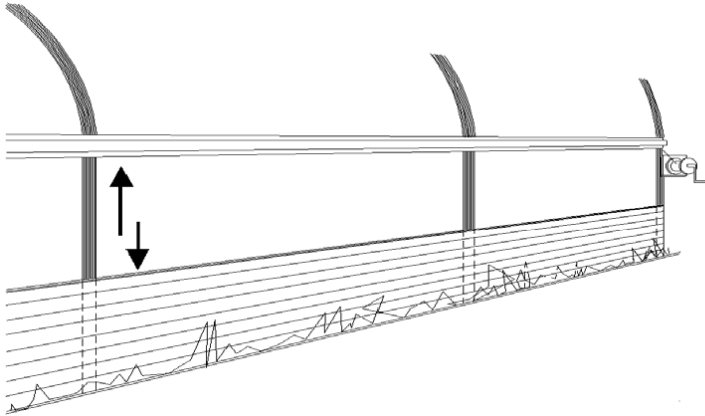
Figure 11 : Ventilation par enroulement de la paroi latérale sur la partie verticale de la coque
