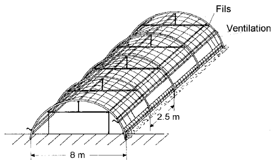
Figure 8 : Tunnel de film plastique avec coupe transversale et ventilation latérale par enrroulement (pratiqué également dans le bi-tunnel)
