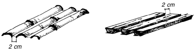
Figure 16: Deux types de sols à claire-voie : en bambou et en poutres en bois
