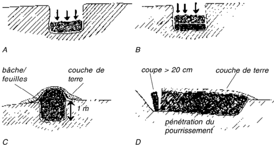
Figure 11: A : On met en place la première couche et on la tasse B : On ajoute une deuxième couche sur la première et on la tasse également. C : La fosse est remplie et couverte hermétiquement D : La fosse est ouverte, l'air peut y pénétrer.
