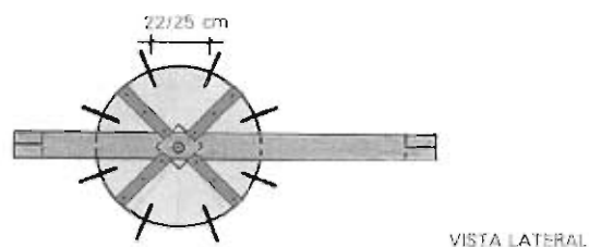
FIG. 8. Vista lateral do rolo-faca com as chapas de fixação dos eixos.
