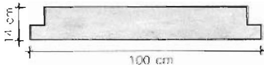
FIG. 1. Uma faca de aço já cortada: a parte que ficou mais larga será encaixada nos sulcos do rolo; no lado oposto, que vai ficar para fora do rolo, a faca recebe um fio bem afiado.
