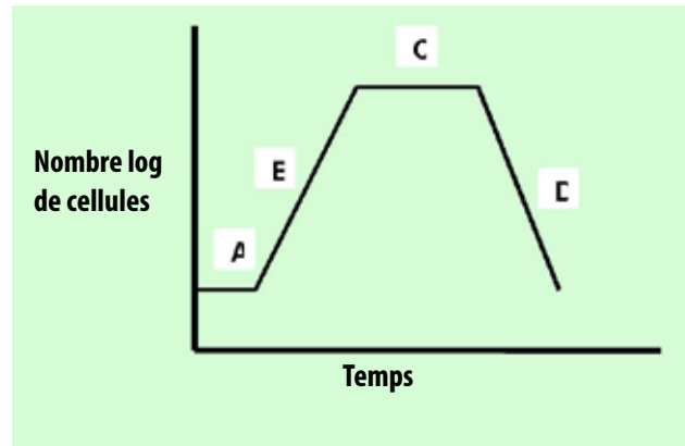
Figure : Courbe-type de croissance de bactéries en culture en batch.
