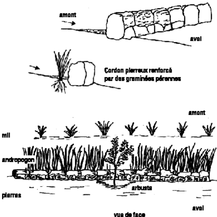
► Figure 2 : Détails d'un cordon pierreux
