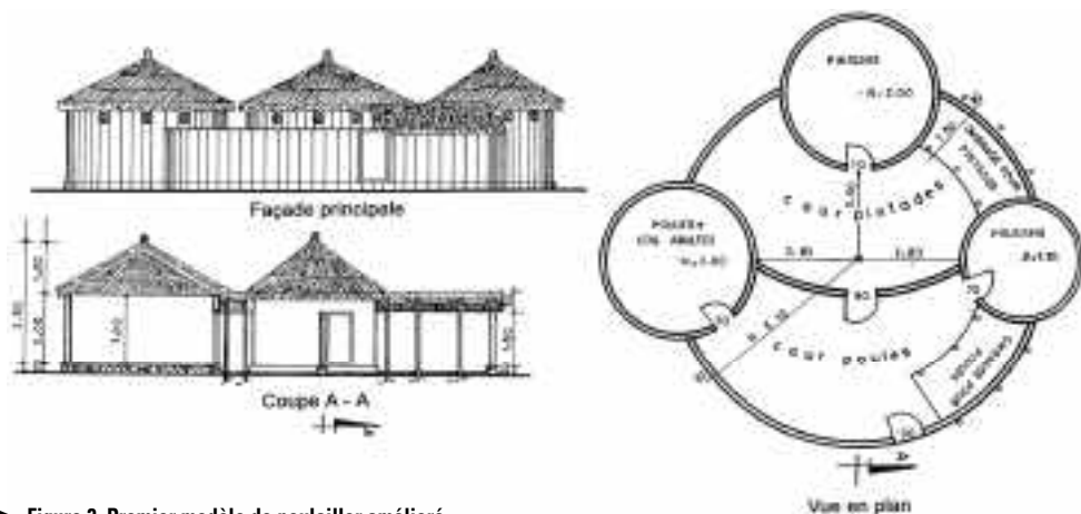
► Figure 3. Premier modèle de poulailler amélioré
