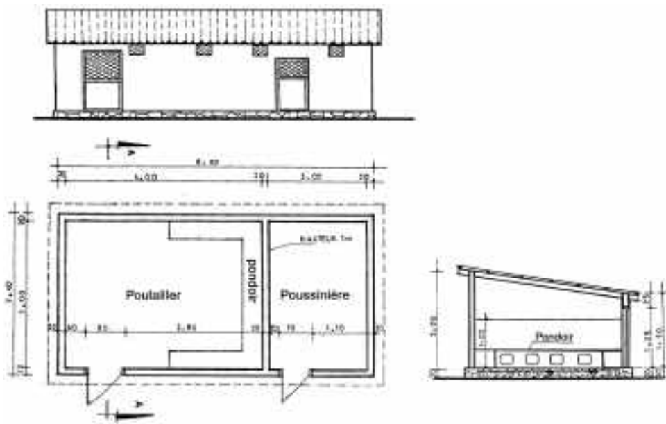
► Figure 4. Second modèle de poulailler amélioré
