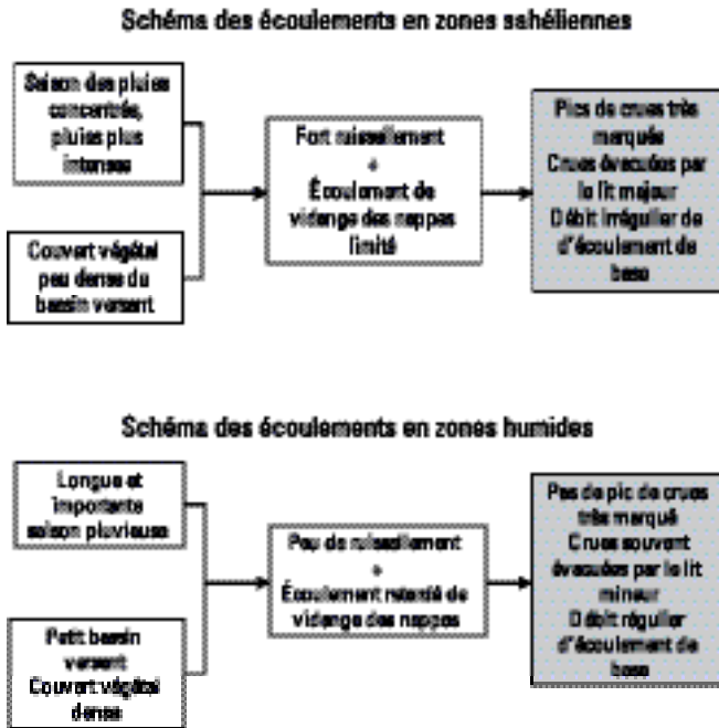
➤ Figure 5 : Ecoulements selon les zones agro-climatiques (Legoupil)
