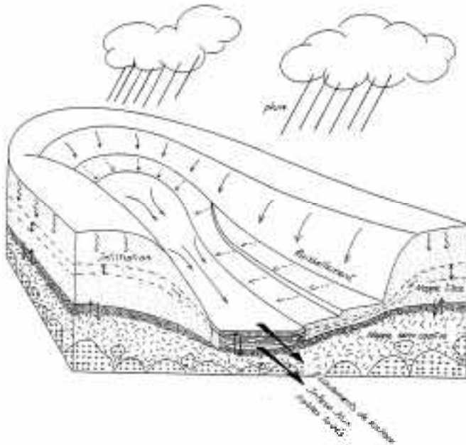
► Figure 2 : Fonctionnement hydrologique d'un bas-fond (Legoupil et al, 2001)
