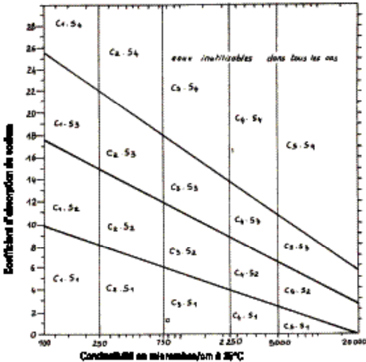
► Figure 1 : Salinité et teneur en sodium des eaux d'irrigation
