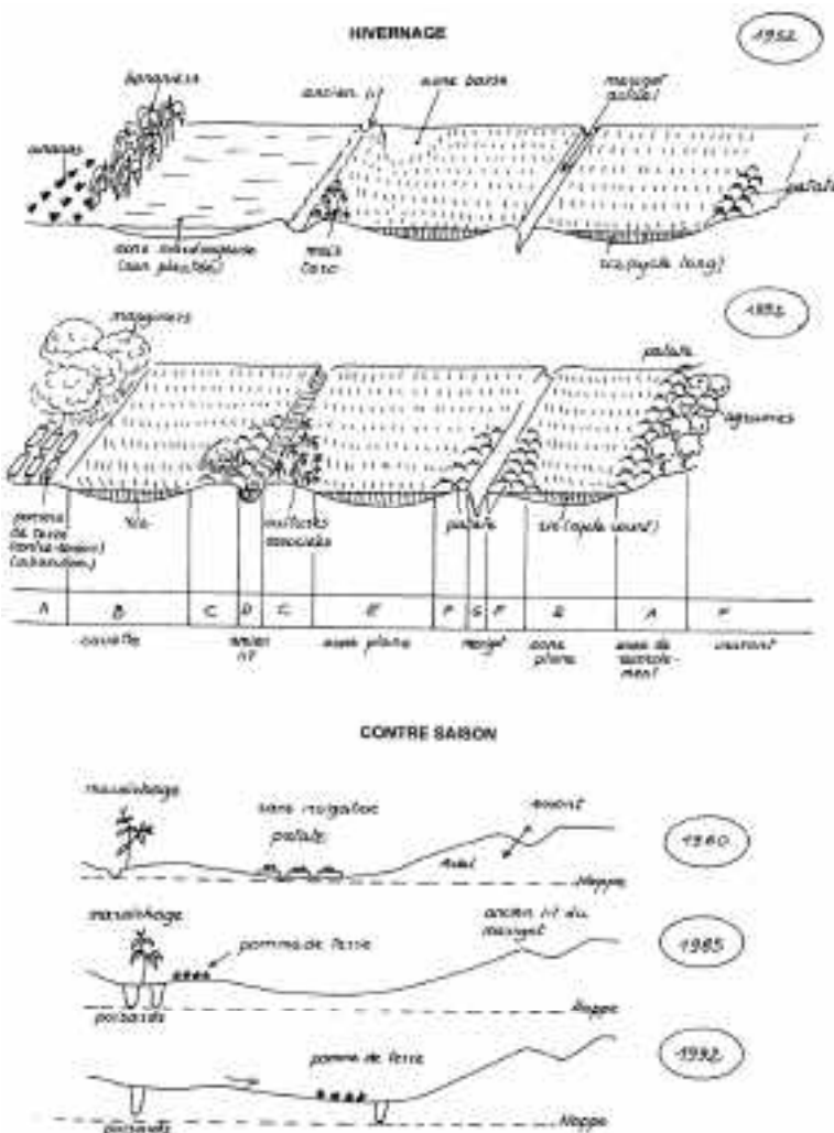
► Figure 8 : Localisation et dynamique des cultures dans le bas-fond de M'Péniasso (Hourdillie, 1993)
