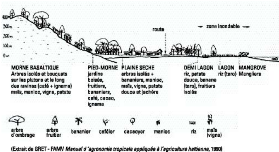
► Figure 4 : Exemple de transect : la région de Camp-Louise en Haïti
