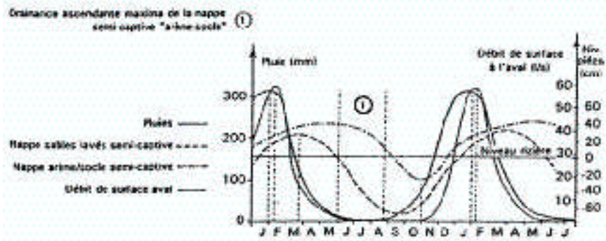
► Figure 3 : Dynamique des nappes à Ambohitrakoho (Raunet, 1993)
