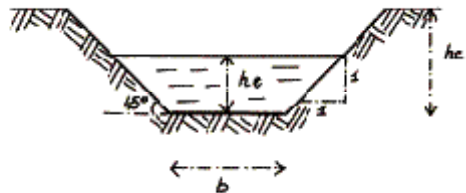
► Figure 2 : Calcul de la forme et la pente des canaux en fonction du débit désiré
