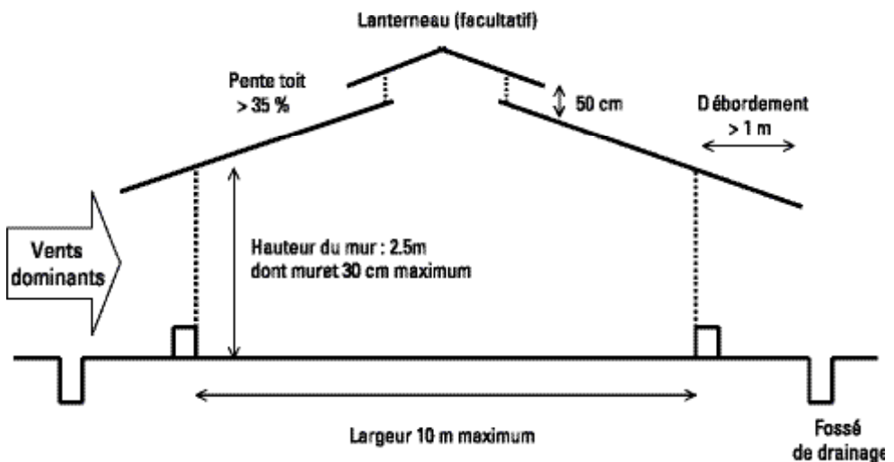
➤ Figure 1. Exemple d'un bâtiment de type ouvert avec toit à deux pentes
