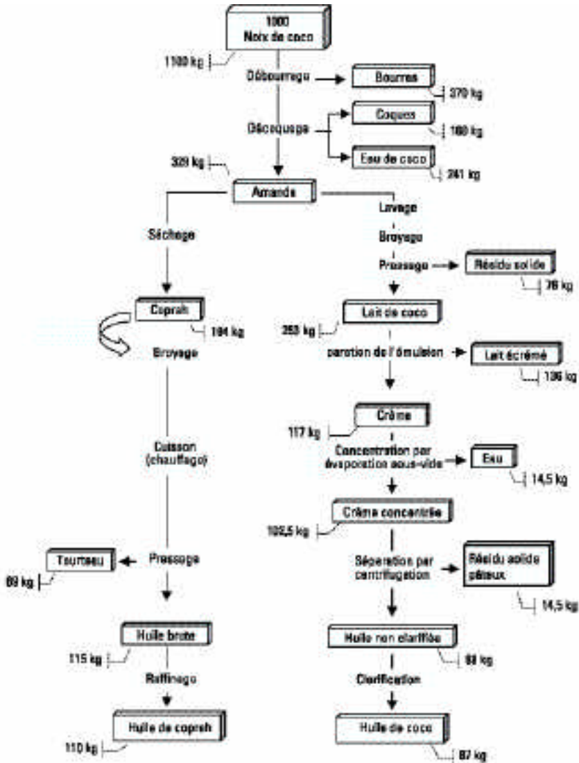
► Figure 2. Les deux types d'extraction de l'huile de coco
