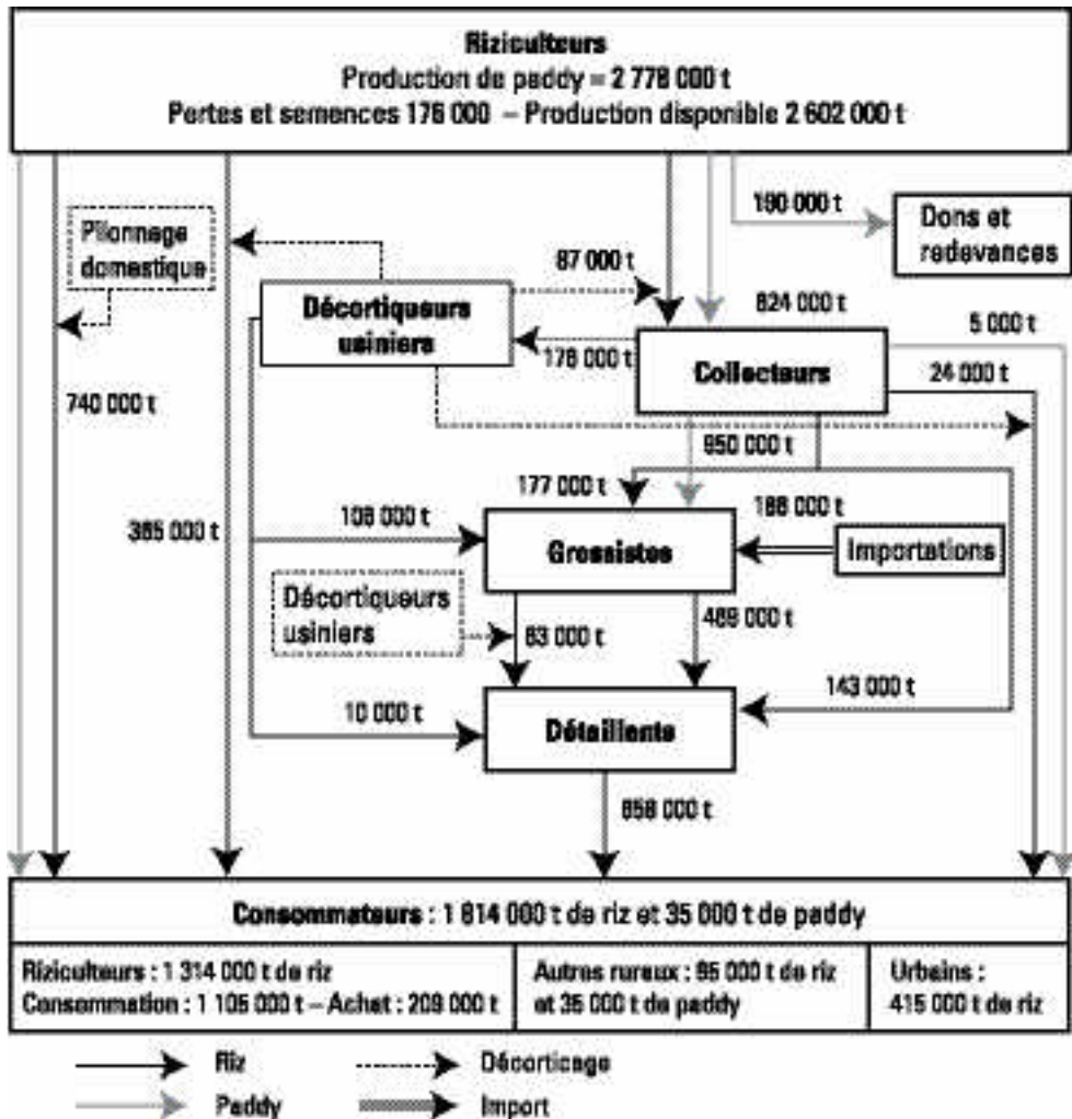
Figure 1: Graphe de la filière riz à Madagascar en 1999
