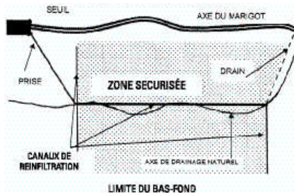
► Figure 12 : Epandage de crues et soutien à la nappe (Lidon et al, 1998)
