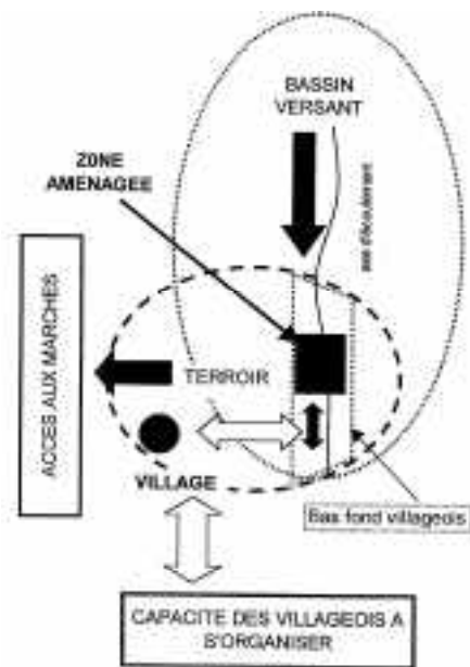
► Figure 7 : Place du bas-fond dans un terroir (Lidon et al, 1998)
