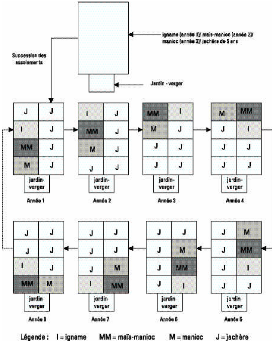
► Figure 2 : Schéma théorique de correspondance entre systèmes de culture et assolement de l'exploitation
