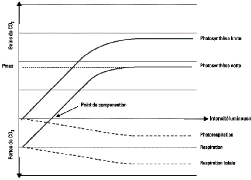
► Figure 4 : Réponse photosynthétique d'une feuille à l'éclaircissement
