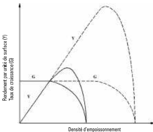
► Figure 2. Présentation schématique des relations entre la densité d'empeusement, le taux de croissance instantané (G), et le rendement instantané par unité de surface (Y), avec (pointillé) et sans (trait plein) alimentation complémentaire (d'après Hepher, 1988, redessiné)
