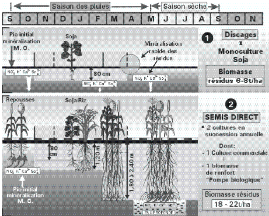
► Figure 5. Effet comparé du travail du sol et du semis direct sur couvertures végétales sur le bilan hydrique et minéral (d'après L. Séguy)
