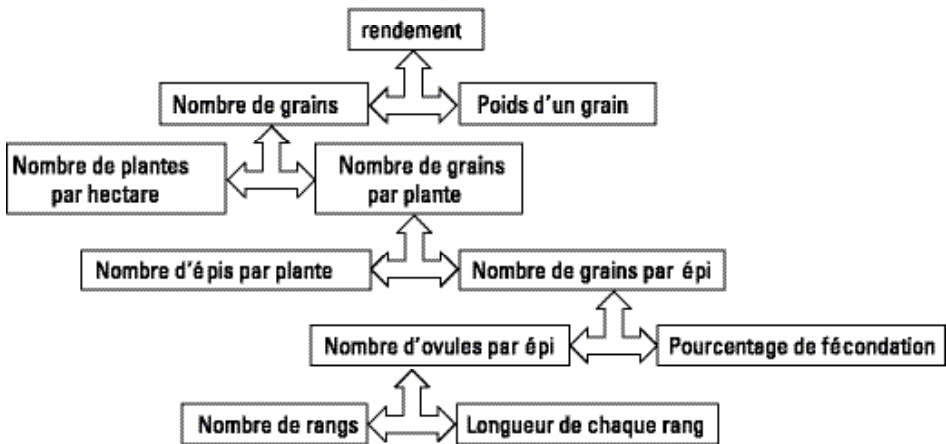
► Figure 1 : Schéma d'élaboration du maïs
