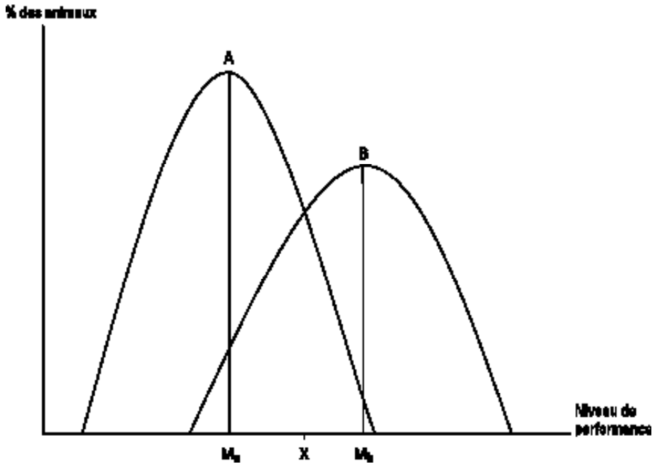
► Figure 1 : Distribution schématique des performances (gain moyen quotidien, par exemple) pour deux populations A (Taurins Baoulé) et B (Zébus)
