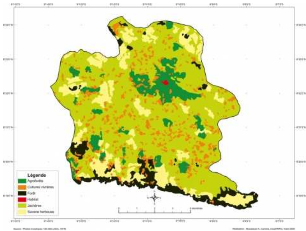
Figure 3 : Évolution de l'occupation des sols à Boussédou (Guinée forestière) entre 1979 et 2008
