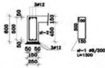
SEC.A-A Scale: 1:25
