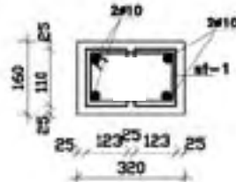
SEC.A-A Scale: 1:10
