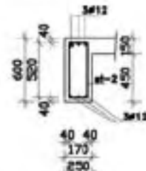
SEC.A-A Scale: 1:25
