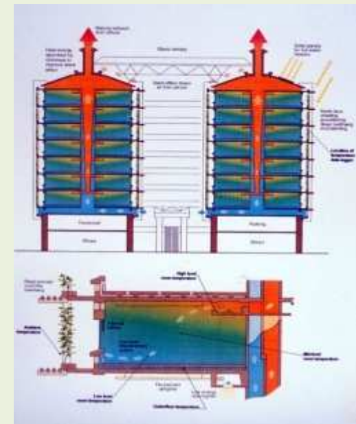
L'Eastgate Centre à Harare, au Zimbabwe, reproduit les structures de ventilation verticales des termitières.
