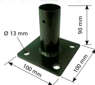
Platine à manchonner
