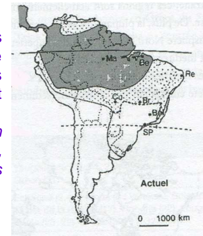
Fig.3 Positions des latérites en Amérique du Sud. En grisé : bauxite; en pointillé : latosols rouges. (D'après Y. Tardy et C. Roquin, ibid ).
