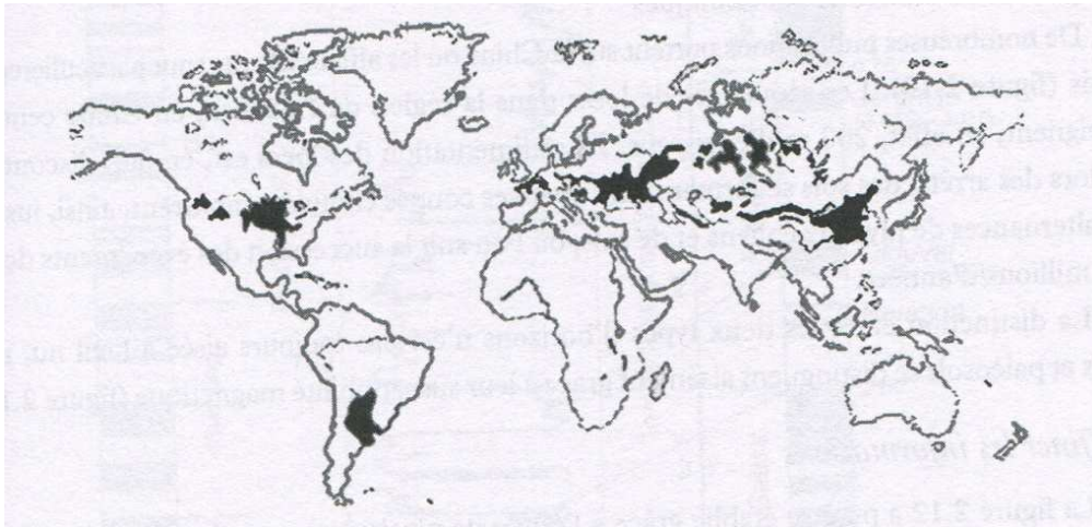
←Fig. 1. Les loess sont bien localisés dans le monde. Dans l'hémisphère Nord, ils se trouvent à des latitudes de l'ordre de 30 à 50°. (D'après Heller et Evans, Loess magnetism , Rev. Geophys., 33, 211240, 1995).
