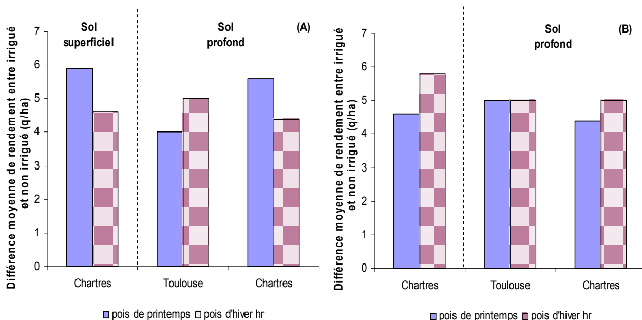
Figure III.6. Ecart de rendement moyen sur 28 climats entre irrigué et non irrigué ( \text{q ha}^{-1} ) pour trois milieux : Chartres en sol superficiel et profond et Toulouse en sol profond en fonction du type de pois et de la précocité au semis (semis précoce (A) et tardif (B)).
