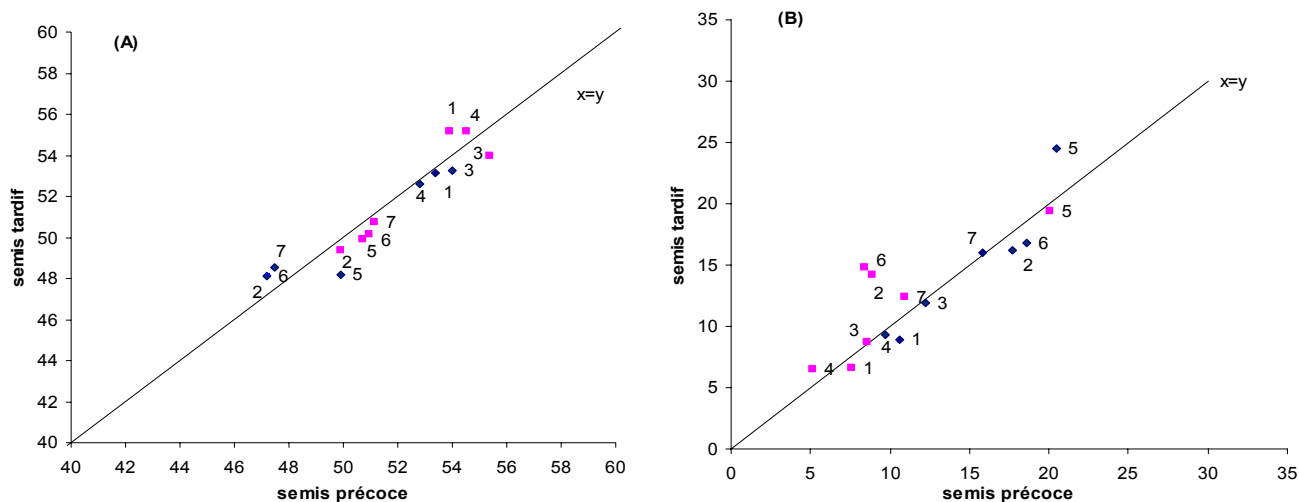
Figure III.3. Confrontation des valeurs simulées de rendement (en q\ ha^{-1} , A) et coefficient de variation (en %, B) en semis précoce et tardif pour les pois de type printemps (◆) et de type hiver (■). Les milieux correspondants (décrits dans le Tableau III.2) sont indiqués par les numéros à côté de chaque symbole.
