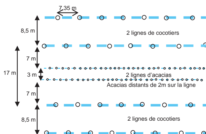
Figure 13. Schéma du dispositif de plantation
